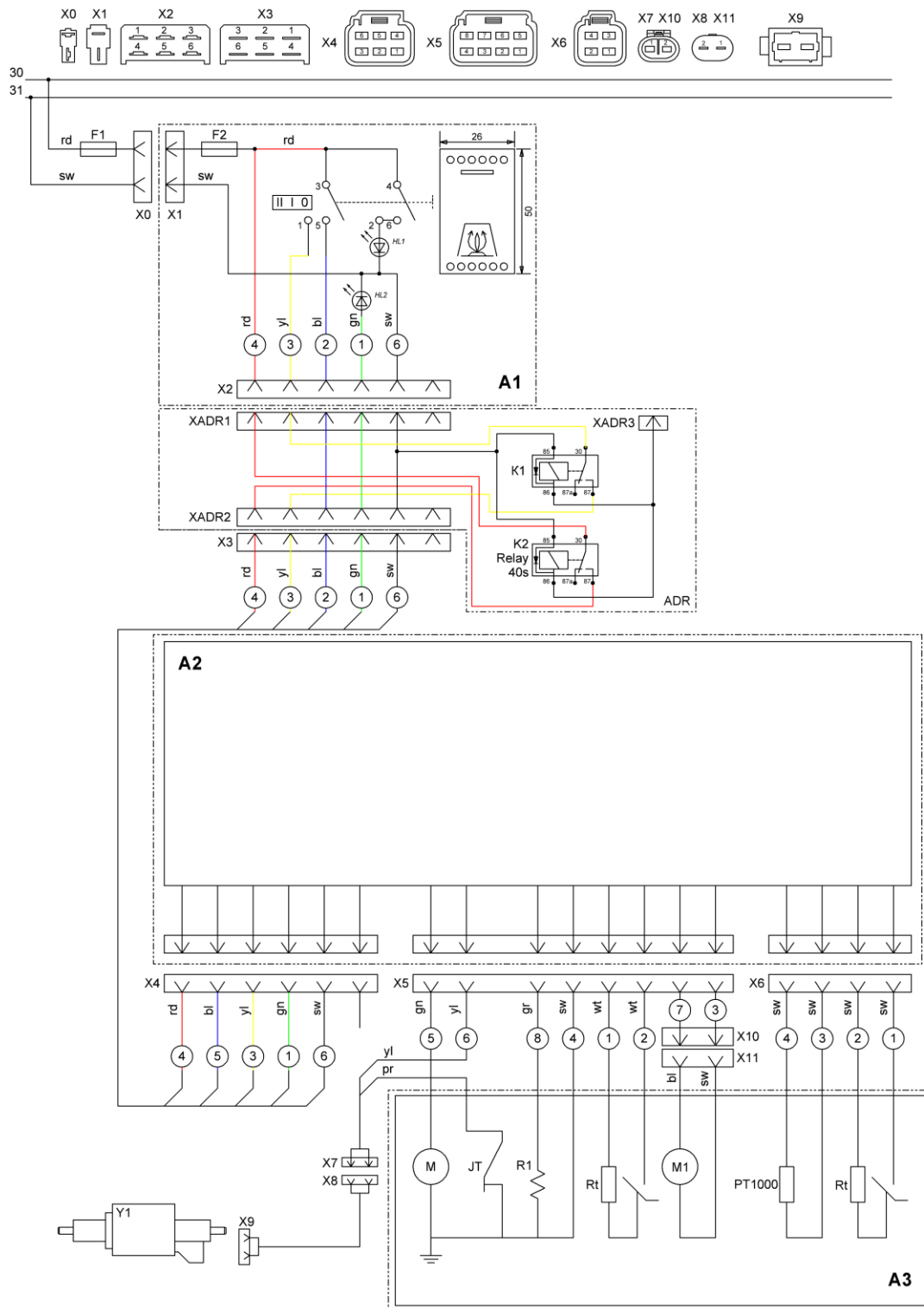
Рис.18 Электрическая схема с функцией ДОПОГ (ADR)
