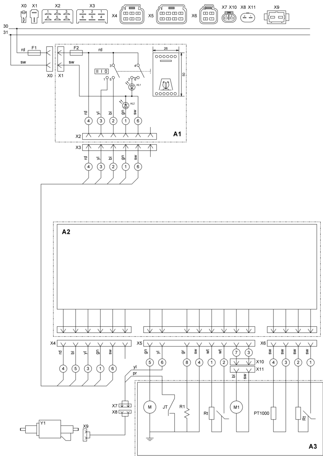
Рис.16 Электрическая схема
