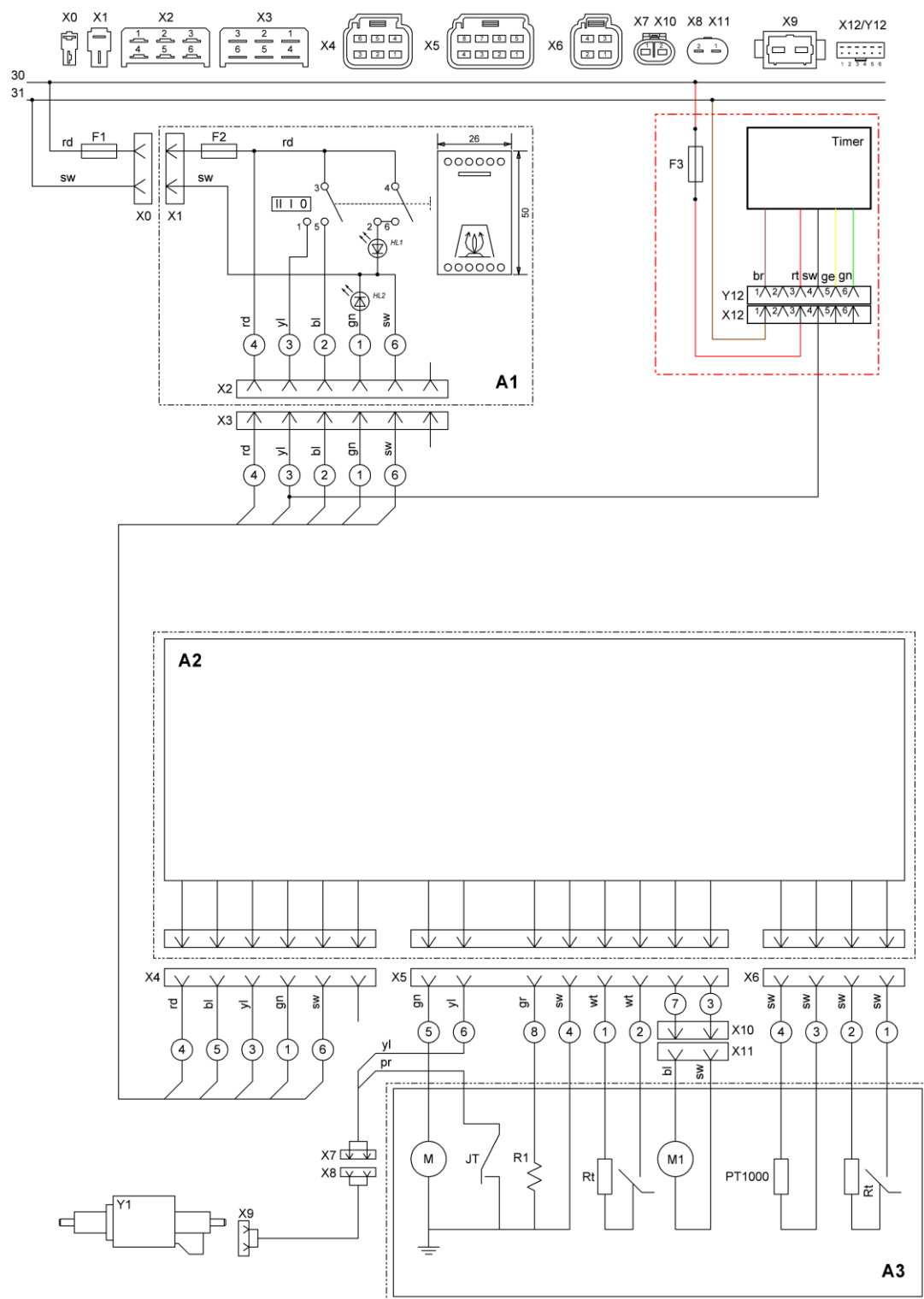
Рис.17 Электрическая схема с Таймером
