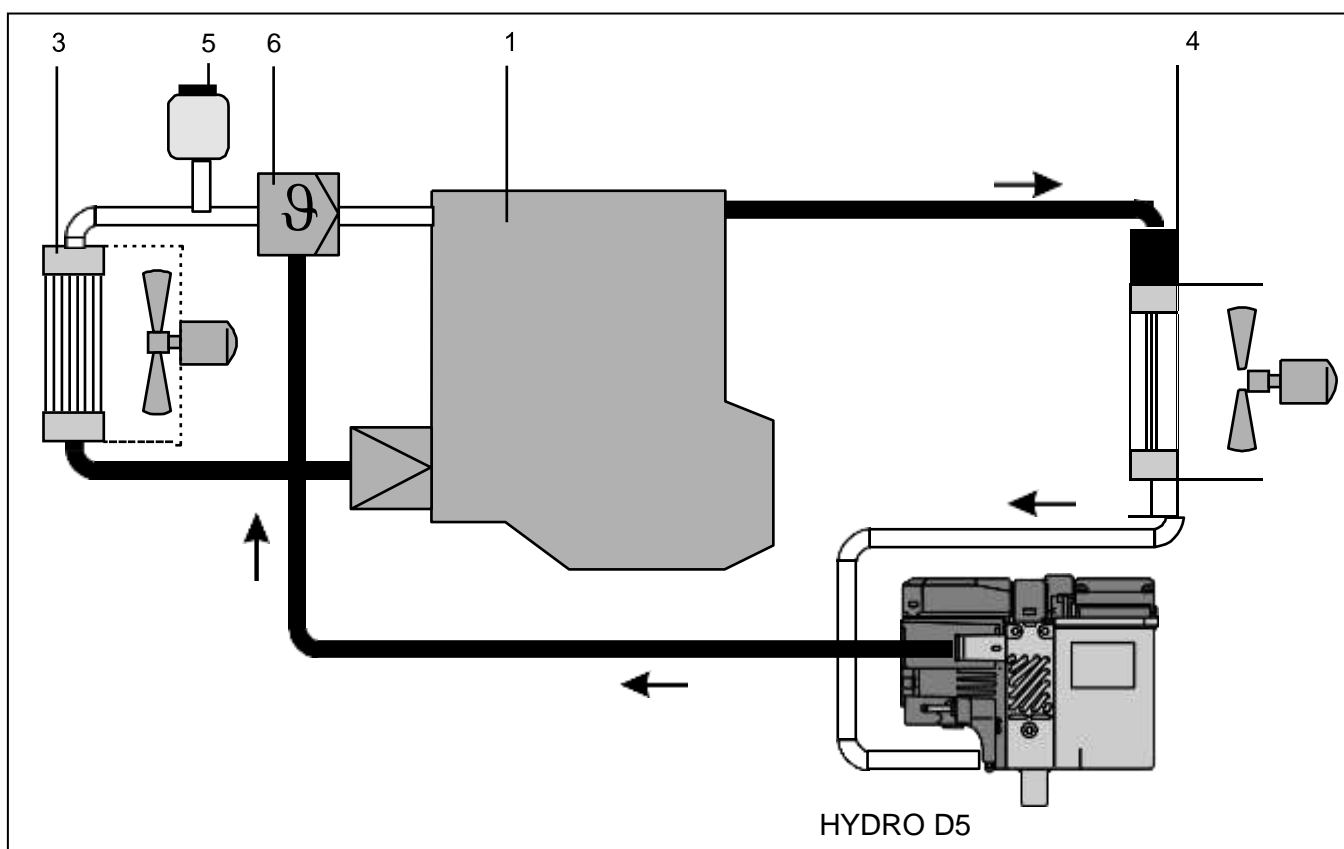
Рис. 7 Установка для преимущественного прогрева двигателя автомобиля
