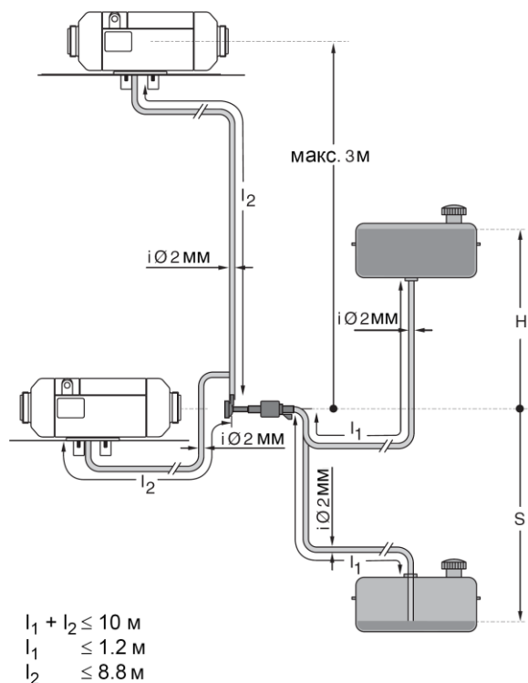
Рис. 801 Система подачи топлива
