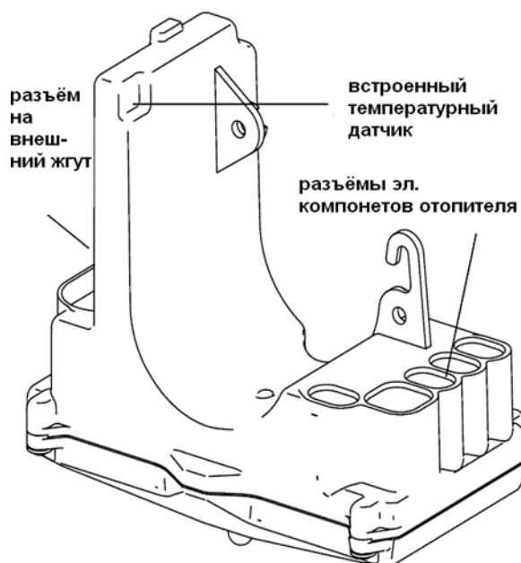
Блок управления
